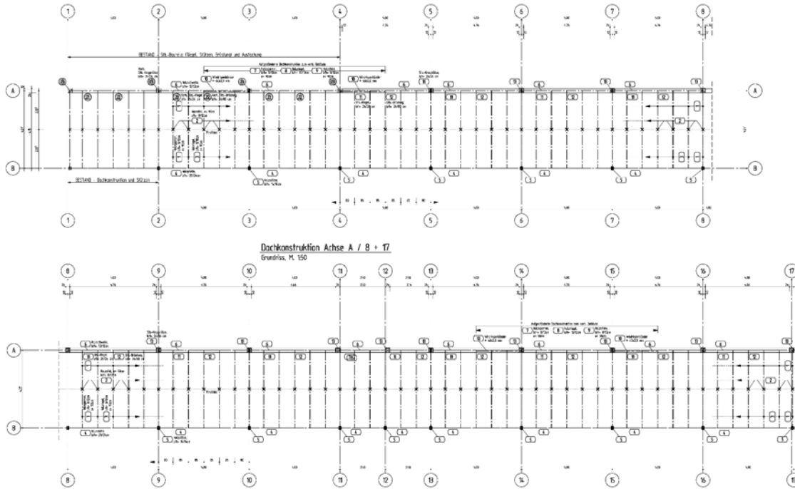
Dachkonstruktion Achse A / 1 + 8 Grundriss, M. 1:50
